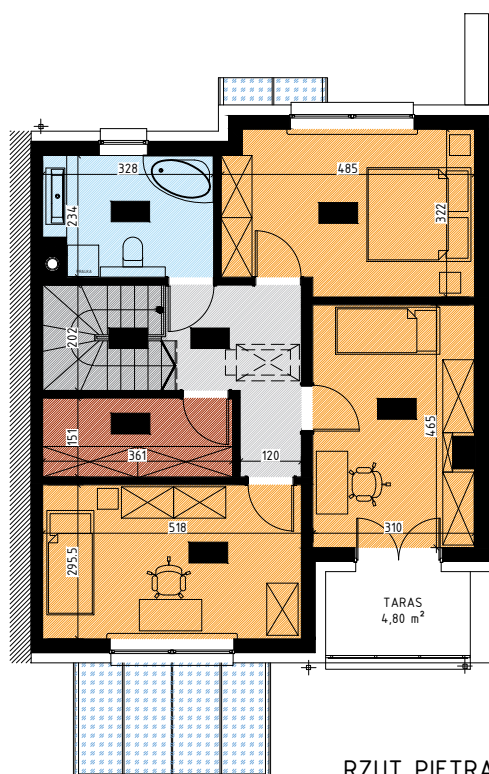
RZUT PIĘTRA
