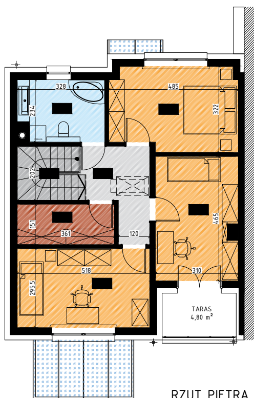
RZUT PIĘTRA
