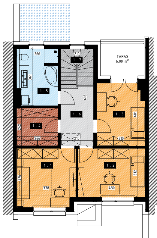
RZUT PIĘTRA
