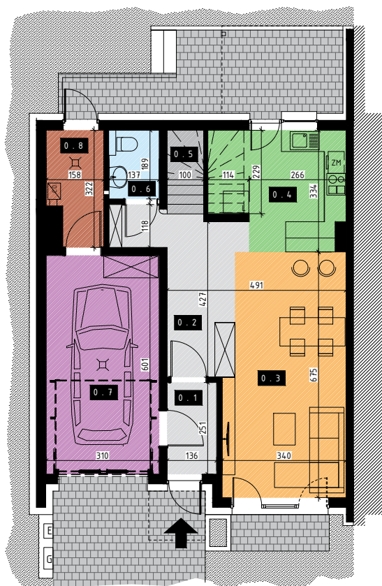
RZUT PARTERU
