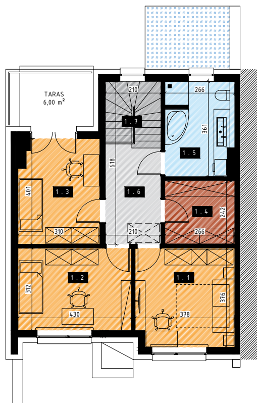
RZUT PIĘTRA
